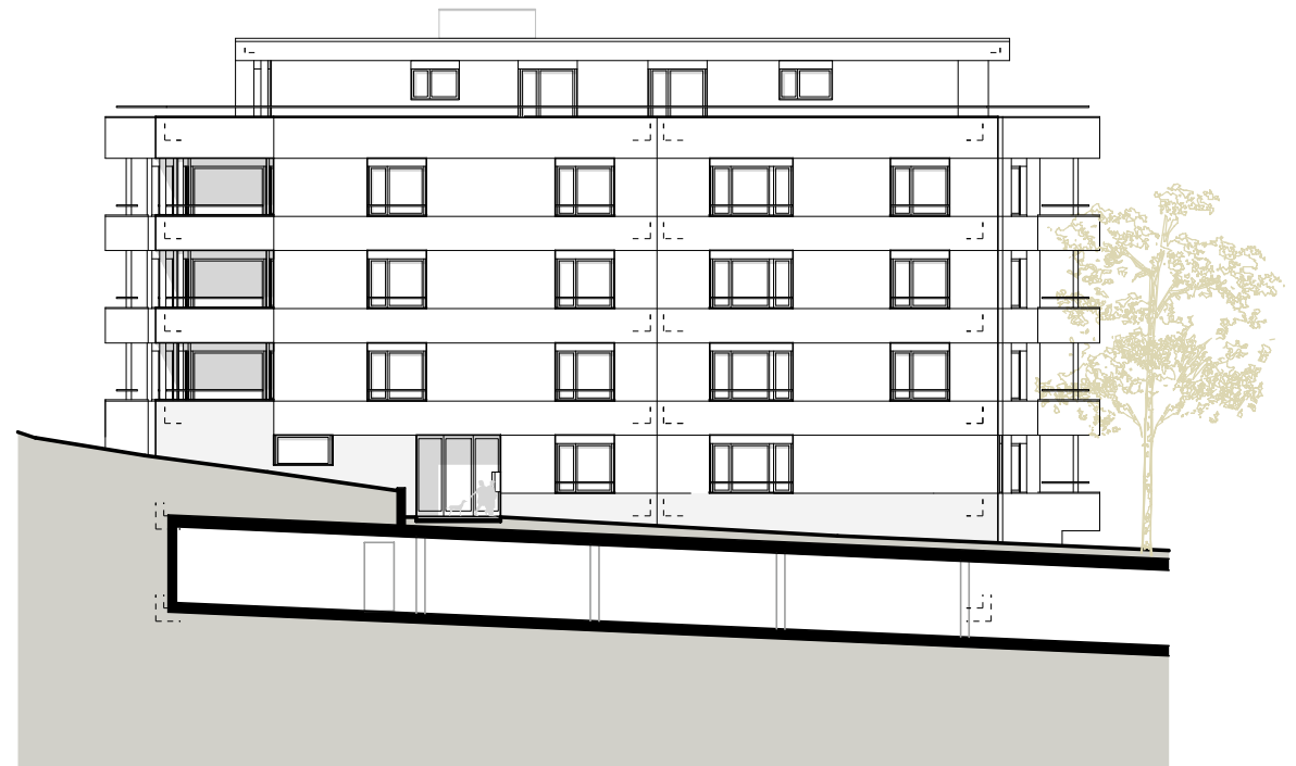
OSTFASSADE
