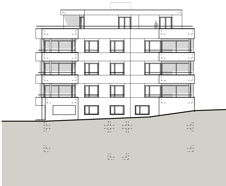
SÜDFASSADE
